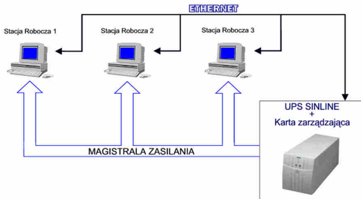
Rys. 11 Przykładowa implementacja scentralizowanego systemu zarządzania zasilaniem przy wykorzystaniu karty zarządzającej SNMP/HTTP
