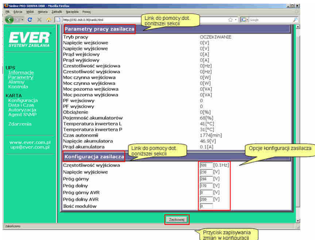
Rys. 6 Przykładowy ekran parametrów zasilacza
