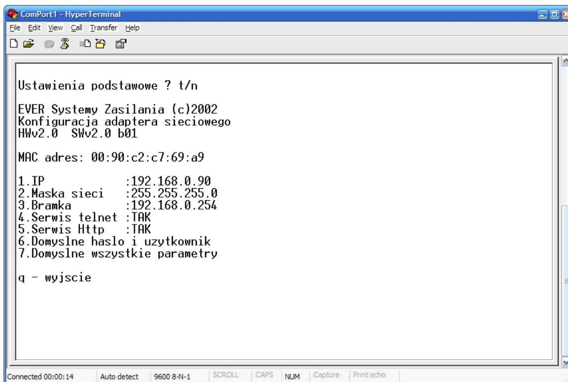
Rys.2 Ekran konfiguracji startowej w aplikacji Microsoft® HyperTerminal
